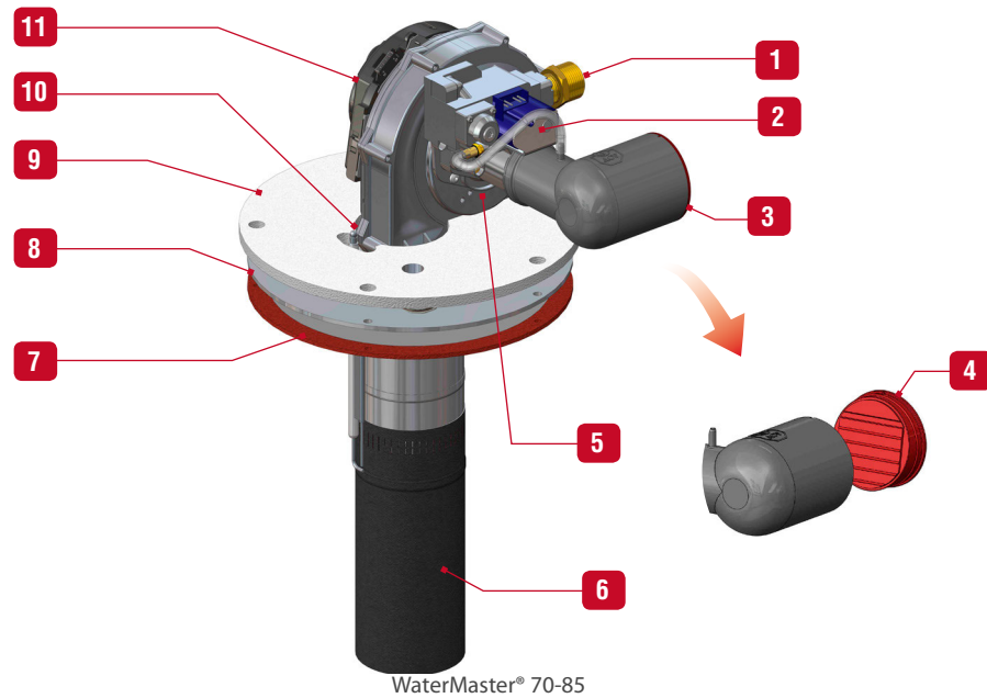
WaterMaster® 70-85
