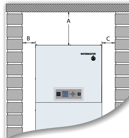
Vooranzicht
