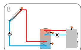
Zonne-energiesysteem met 1 boiler en vaste brandstofketel (pagina 16)
