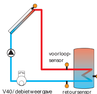
V40/ debietweergave retoursensor
