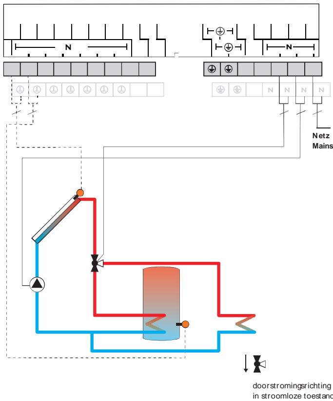
Display weergave Systeem 10
