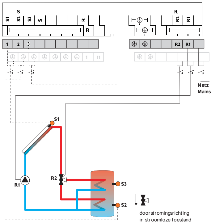
Display weergave System 4
